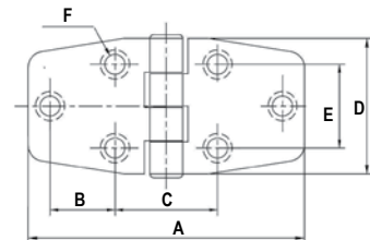
Hinge, Inox 316
