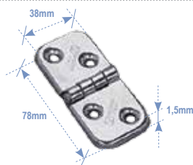
Hinge, Inox 316
