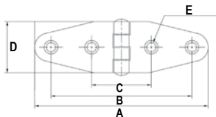
Hinge, Inox 316
