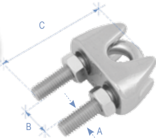
Wire Rope Clip
