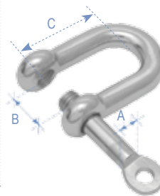
Ναυτικό Κλειδί, Τύπου D, με Πείρο που Κλειδώνει, AISI 316
