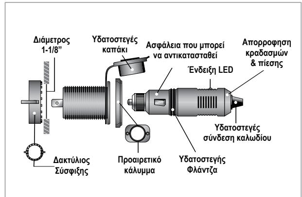
Πρίζα Ρευματολήπτη, 12V
