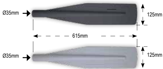
Παλάμη για τα Κουπιιά 50992-50995
