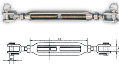
Εντατήρας Ανοικτού Τύπου, Jaw & Jaw, Inox 316
