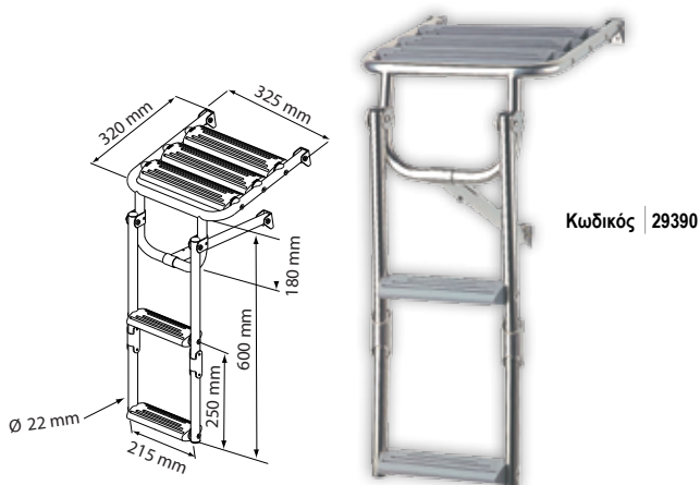
Σκάλα Inox 316 με Πλατφόρμα & 2 Πλαστικά Σκαλιά
