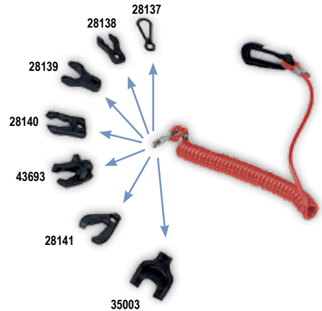
Κλειδί Kill Switch με Σπιράλ, Σετ
