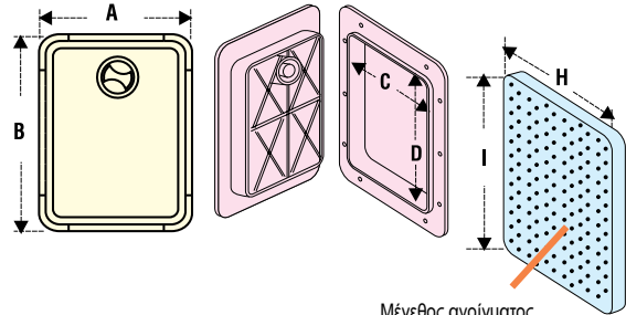
Μέγεθος ανοίγματος στο κατάστρωμα για εγκατάσταση.
