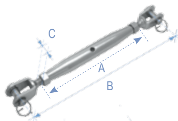
Εντατήρας Κλειστού Τύπου, Jaw & Jaw, Inox 316
