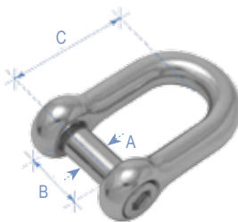
Ναυτικό Κλειδί, Τύπου D, με Εσωτ. Εξαγωνικό Πείρο, AISI 316
