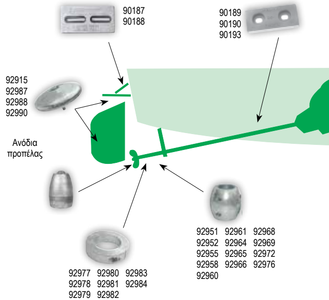
Ανόδια για Χρήση σε Εσωλέμβιες Μηχανές
