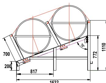
Βάση για SOLAS OCEANO, 2 θέσεων, 30-35(A)
