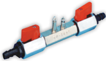
Βαλβίδα Καυσίμου 2 Δρόμων, για Σωλήνα Ø 10 mm
