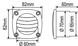
Περσίδα Αεραγωγού, Λευκή
