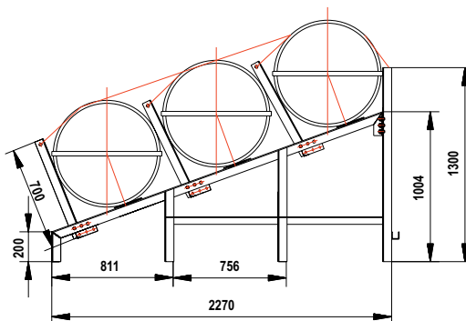
Βάση για SOLAS OCEANO, 3 θέσεων, 6-25(A), 6-35(B)
