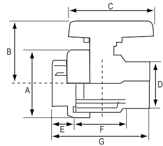
Βαλβίδα Ένσφαιρη, Single Union, BSPP, Πλαστική, με Πορτοκαλί Λαβή
