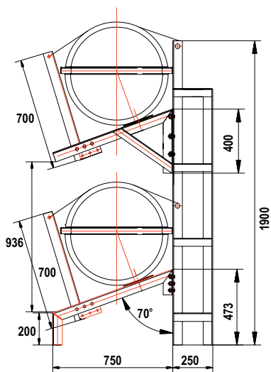
Κάθετη Βάση για SOLAS OCEANO, 2 θέσεων, 6-25(A), 6-35(B)
