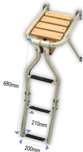
Πλατφόρμα Ξύλινη με Σκάλα Inox 316
