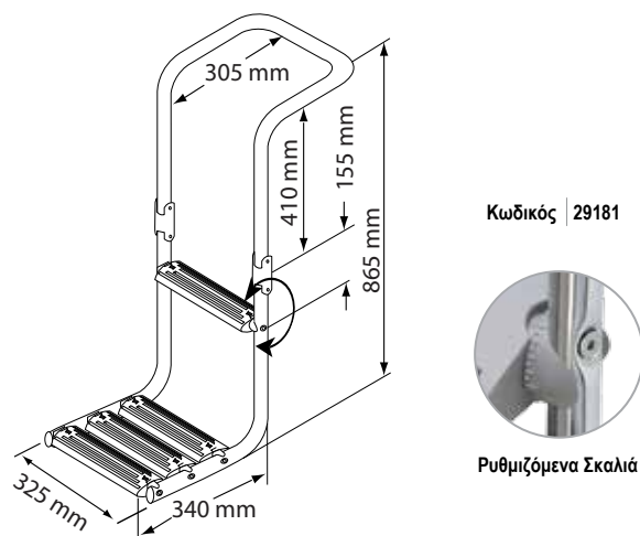
Βυθιζόμενη Σκάλα-Πλατφόρμα, Inox 316
