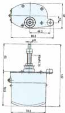
Μοτέρ Υαλοκαθαριστήρων, Inox, 90°
