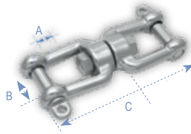
Στριφτάρι με 2 Κλειδιά, Inox 316
