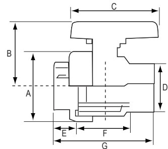
Βαλβίδα Ένσφαιρη, Single Union, BSPP, Πλαστική, με Μπλε Λαβή
