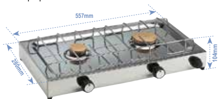
Εστία Γκαζιού, Διπλή Βάρος : 3 kg
