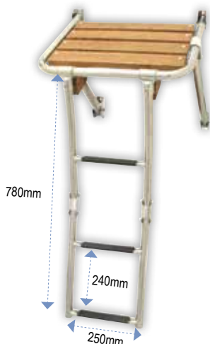
Πλατφόρμα Ξύλινη με Αναδιπλούμενη Σκάλα Inox 316
