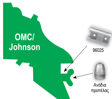
Ανόδιο για Εσω - Εξωλέμβιες Μηχανές OMC/Johnson
